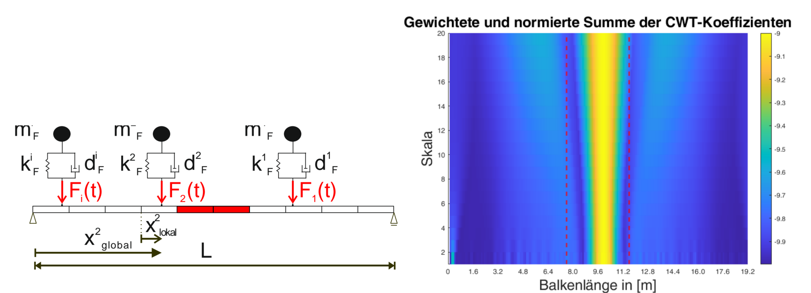
Abbildung 2: links: numerische Simulation der Fußgängerbrücke mit fiktiver Steifigkeitsveränderung in Feldmitte unter Berücksichtigung der passierenden Fußgänger; rechts: Ergebnis der Wavelet-Transformation zur Lokalisierung der Steifigkeitsveränderung
